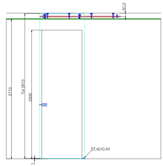
Vereinfachte Darstellung der Vorderansicht, gebogene Schiebetür Simplified representation of front view, curved sliding door
